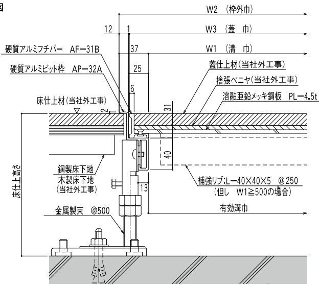
■断面図
