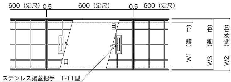
ステンレス揚蓋把手 T-11型
