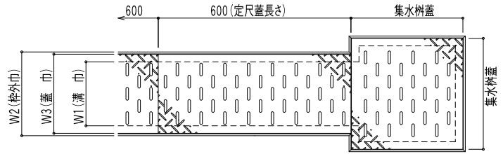
■平面図
