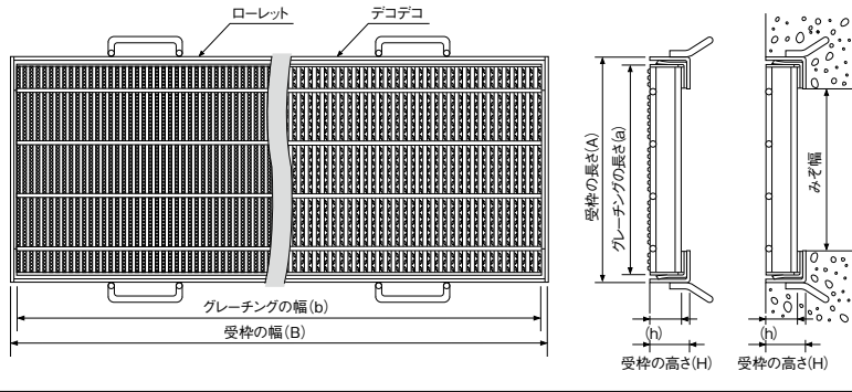
■平面図
