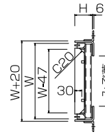
■ピッチ詳細図 9.5 4.5 9
