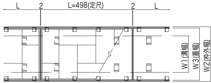
■平面図
