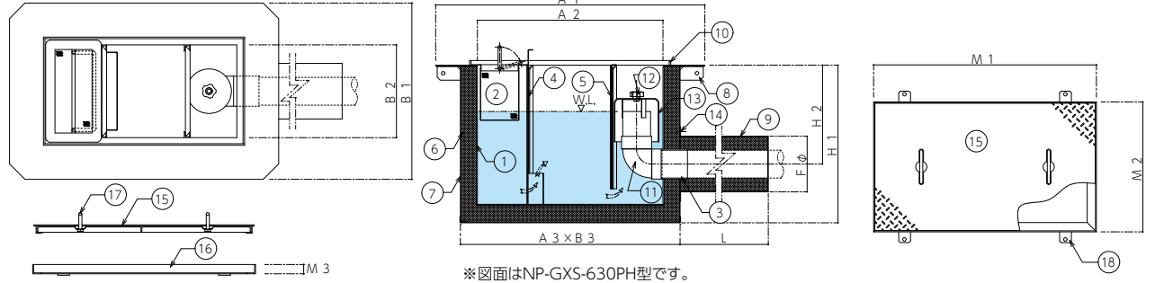
※図面はNP-GXS-630PH型です。
