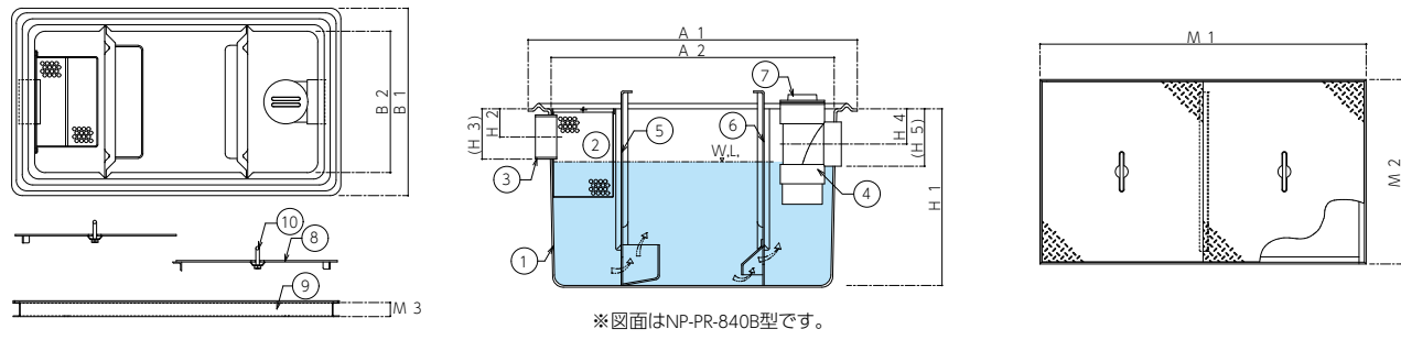
※図面はNP-PR-840B型です。
