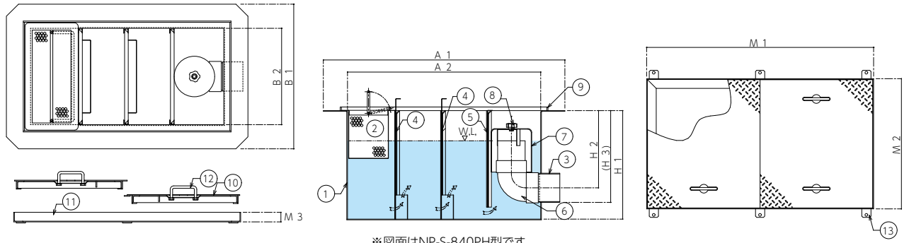
※図面はNP-S-840PH型です。
