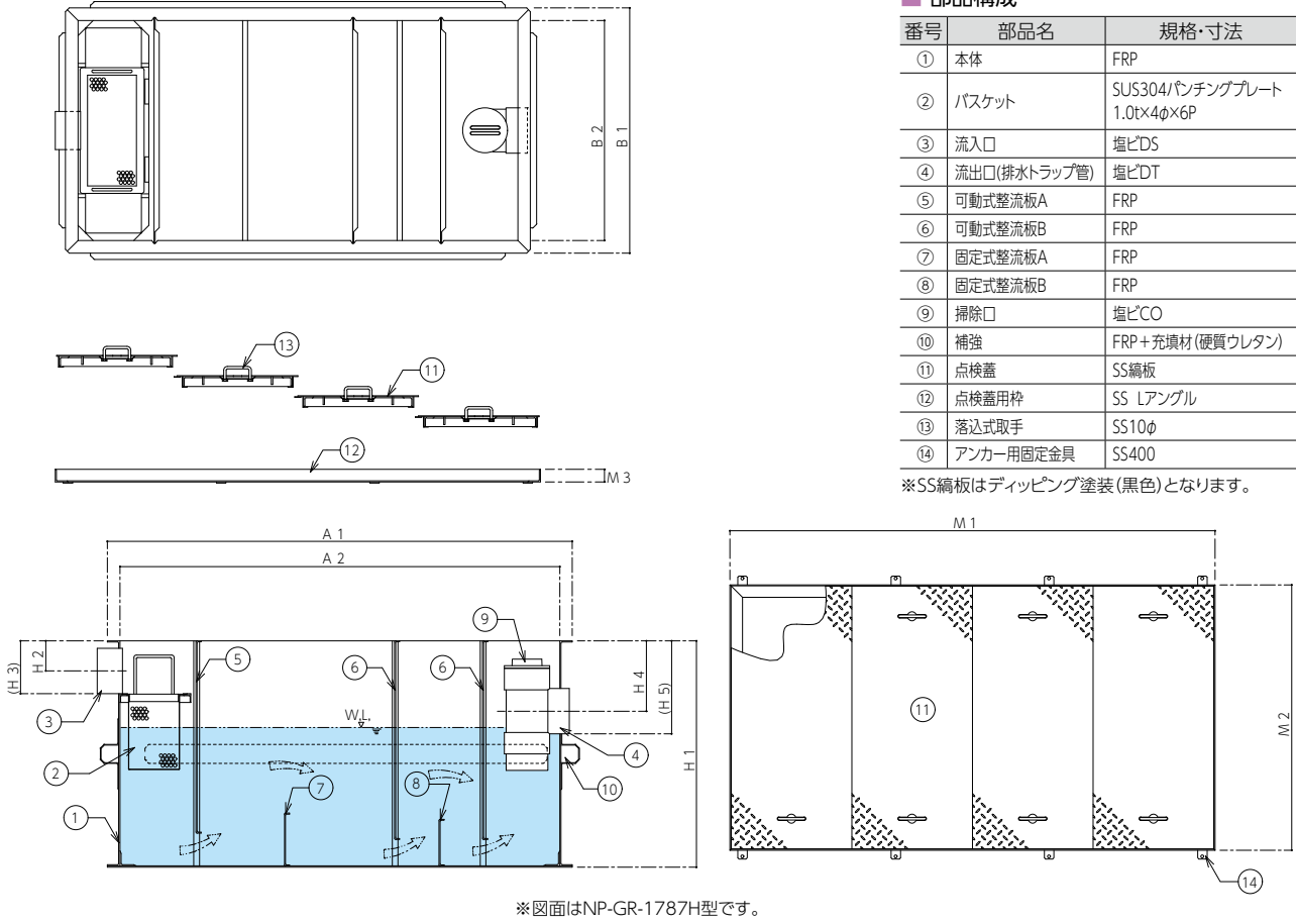
※図面はNP-GR-1787H型です。
