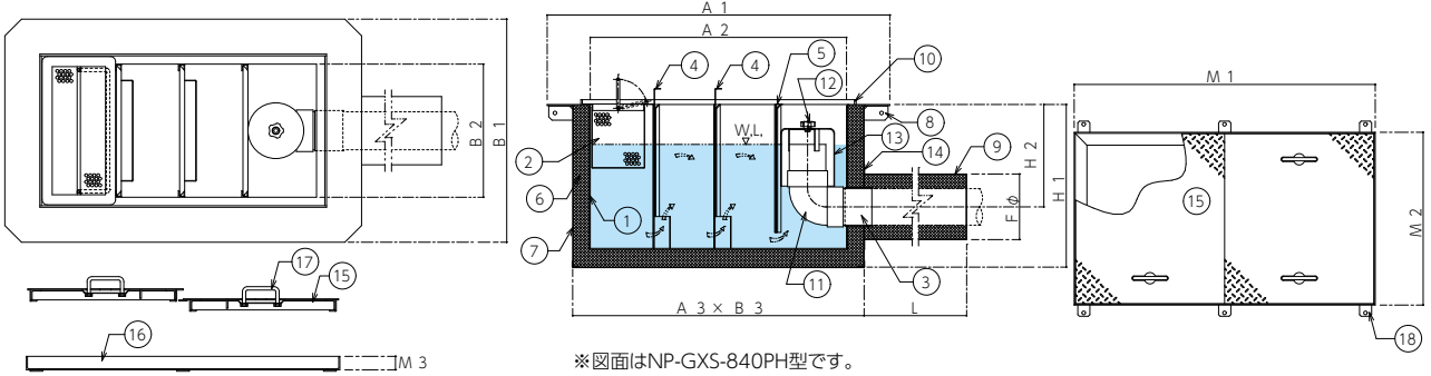
※図面はNP-GXS-840PH型です。
