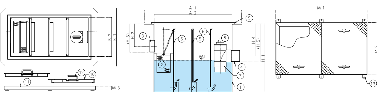
※図面はNP-SR-840H型です。
